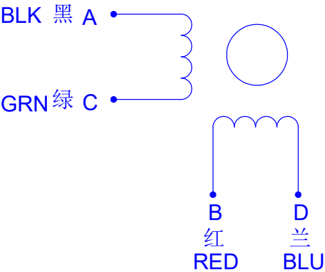
Wiring Diagram:
